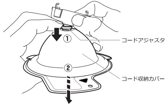
引掛埋込ローゼット (ハンガー付)
