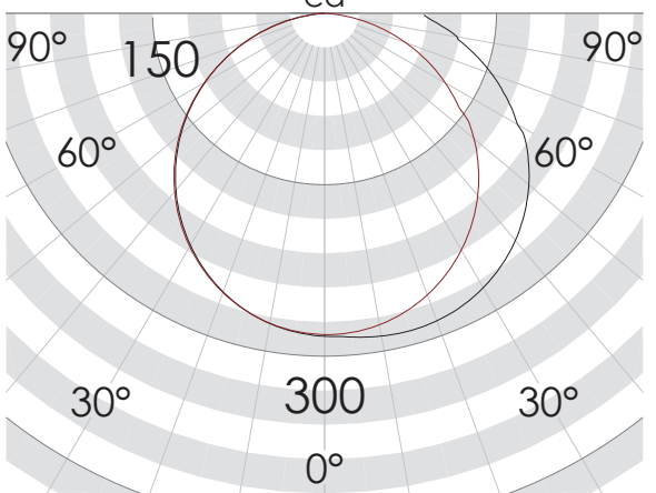
配光曲線
