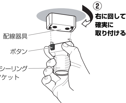
引掛埋込ローゼット (ハンガー付)
